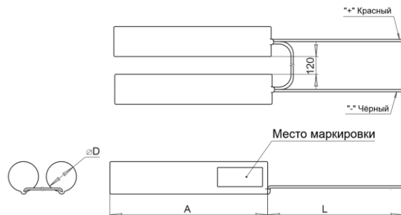
Рис.9 Габаритные размеры BS-3+3KRHT23/43-1.5/L-HB500-0-1 a18268
