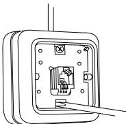
3.5. Закрепить механизм на поверхности при помощи саморезов (в комплект поставки не входят). Защелкнуть крышку.
