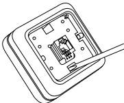
3.2. Отсоединить крышку от задней панели, отжав наконечником отвертки защелки.
