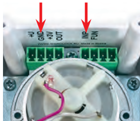
Фото 9. Клеммы подключения проводных датчиков — INP, GND
