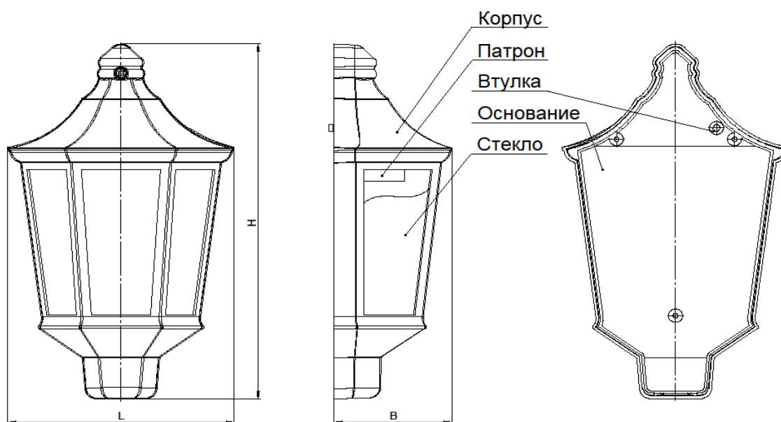
Светильник НБУ 06-60-003 У1 "Ника"
