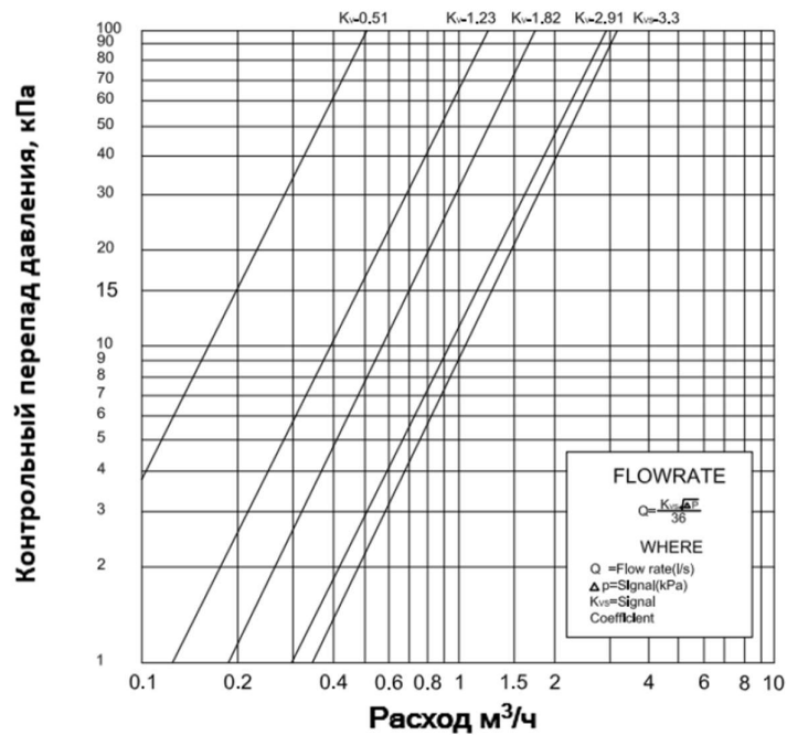
Клапан 1206 DN20
