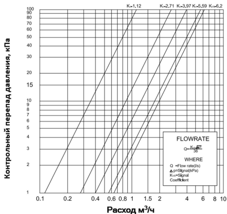
Клапан 1206 DN20
