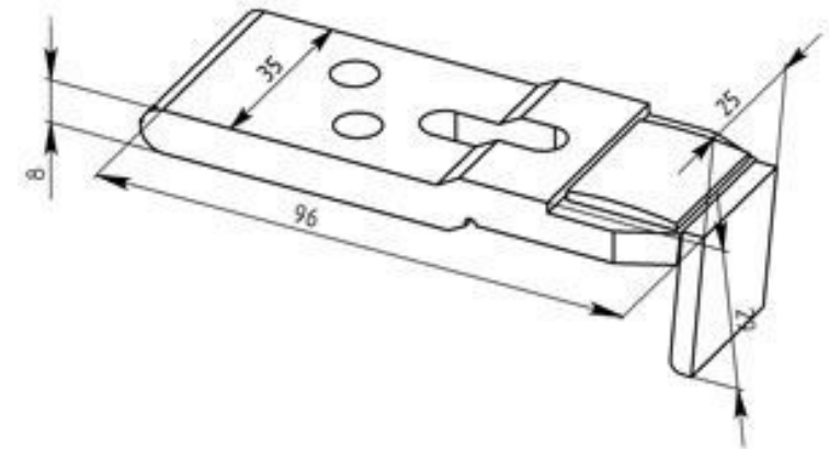
Контакт контактора ES-250 (подвижный)
