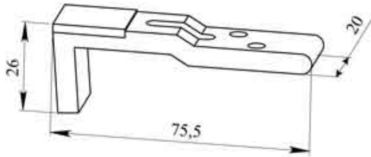
Контакт контактора ES-160 (подвижный)
