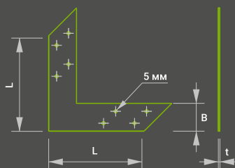
Угловой соединитель US
