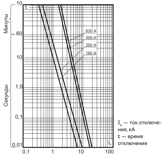
Предохранители типа ПНБ5-380/250, ПНБ5-1250/630
