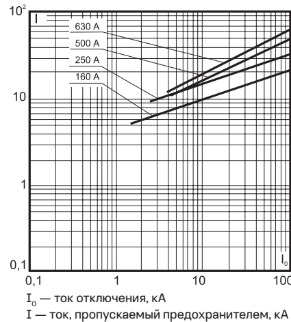
Предохранители типа ПНБ5-380/250, ПНБ5-1250/630
