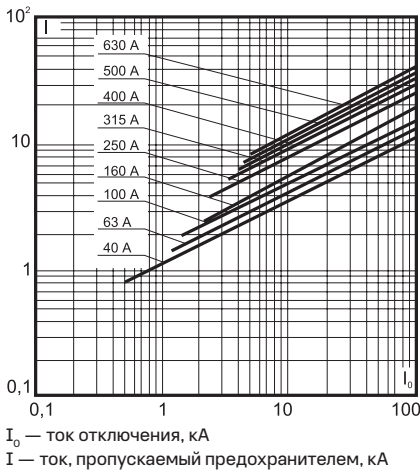
Предохранители типа ПНБ5М-380/400, ПНБМФ-380/400, ПНБ5М-380/630
