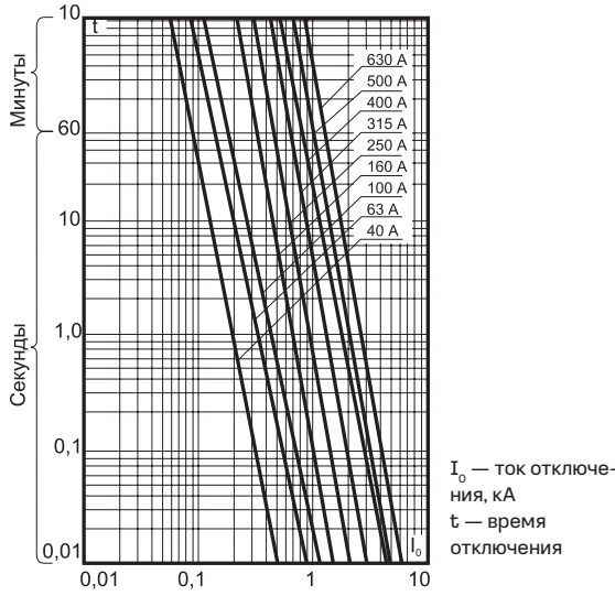
Предохранители типа ПНБ5М-380/400, ПНБМФ-380/400, ПНБ5М-380/630
