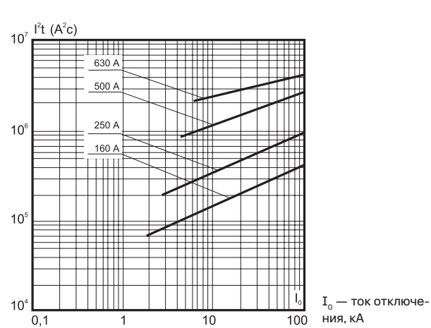
Предохранители типа ПНБ5-380/250, ПНБ5-1250/630
