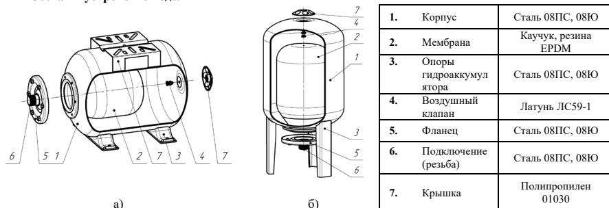
Рисунок 1 – Общий вид и конструкция гидроаккумулятора а) боковое подключение; б) нижнее подключение
