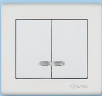
41001023 Выключатель двухклавишный с подсветкой Напряжение 250V Сила тока 10A Степень защиты IP20
