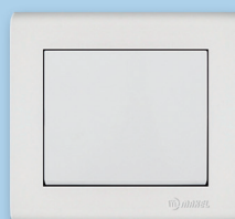
41001020 Переключатель проходной Напряжение 250V Сила тока 10A Степень защиты IP20
