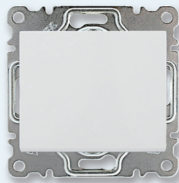
(2A) Механизм с клавишей / панелью
