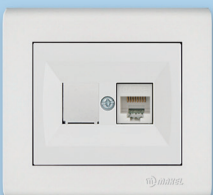
41001035 Розетка комп. двойная (1шт. Cat 5) Степень защиты IP20
