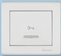
41001097 Кнопка для автоматического открывания двери с подсветкой Напряжение 250V Сила тока 10A Степень защиты IP20
