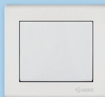
41001095 Выключатель одноклавишный 3 входа 3 выхода Напряжение 250V Сила тока 10A Степень защиты IP20
