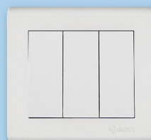
41001091 Выключатель трёхклавишный 1 вход 3 выхода Напряжение 250V Сила тока 10A Степень защиты IP20
