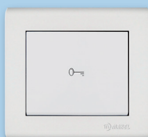
41001096 Кнопка автоматического открывания двери Напряжение 250V Сила тока 10A Степень защиты IP20
