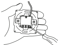
3.4. Присоединить к розетке предварительно зачищенный кабель.
