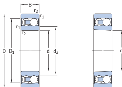
Цилиндрическое отверстие
