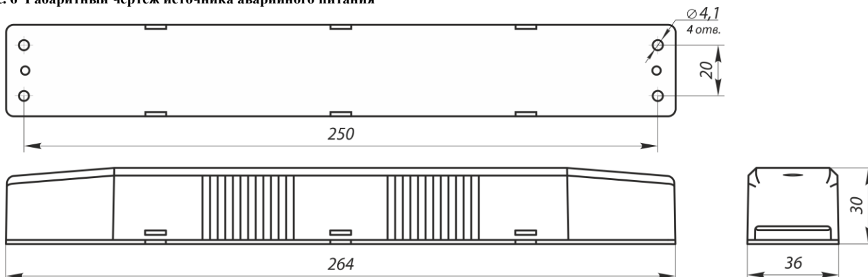
Рис. 6 Габаритный чертеж источника аварийного питания
