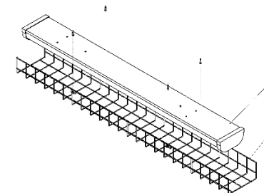
Сурет 1. Қорғаныс торын орнату схемасы
