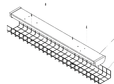
Рисунок 1. Схема монтажа защитной решётки
