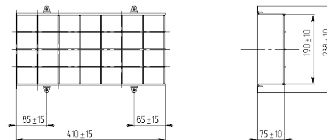
Сурет 1. Қорғаныс торын орнату схемасы
