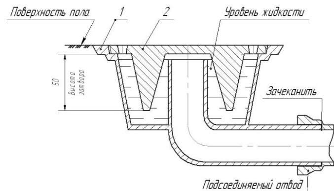
Рис. 2. Схема установки трапа горизонтального – 50/100
