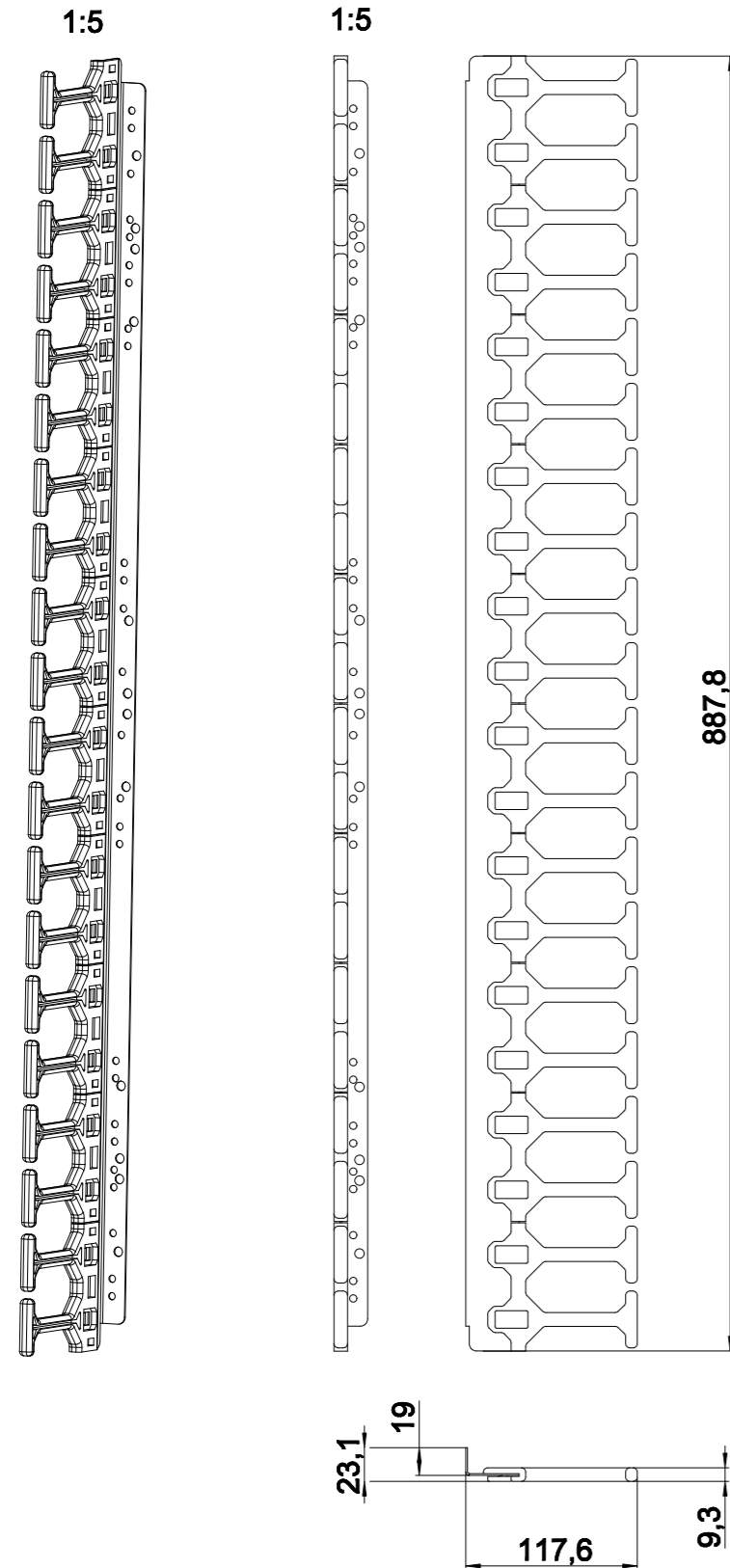
ИДФУ.304403.084-01 Органайзер ВКО-П-20/42U
