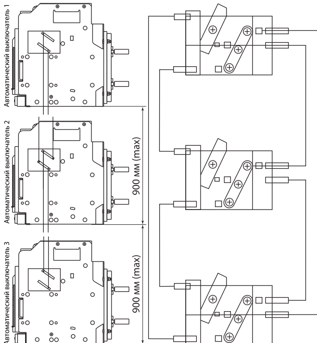
Рисунок 47. Блокировка трех автоматических выключателей
