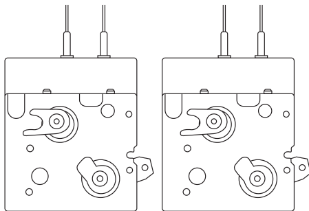
Рисунок 45. Механическая блокировка
