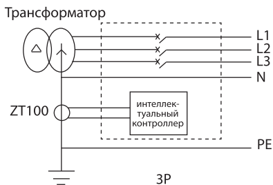
Рисунок 14. Варианты защиты от замыкания на землю и электрические схемы
