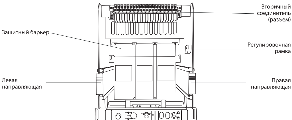
Рисунок 3. Выдвигная панель (седло) выключатель выдвинут и снят (пример ВА90-2000)
