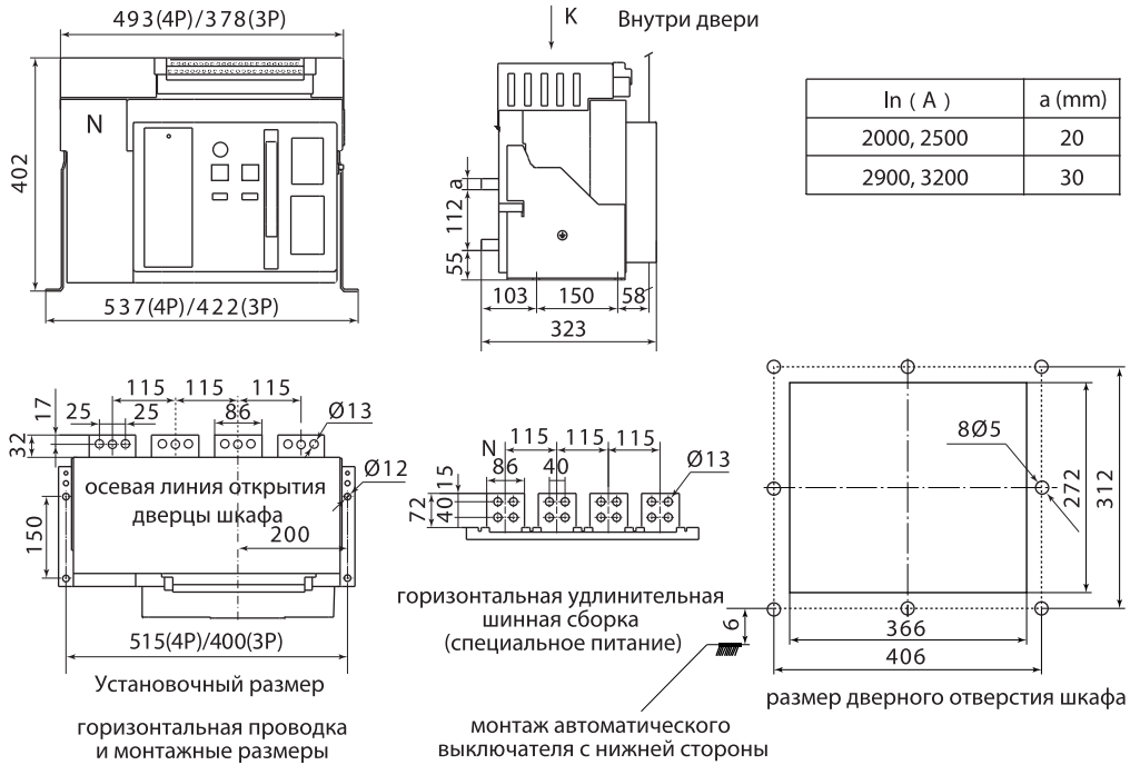
Рисунок 23. Габаритные и установочные размеры ВА90-3200 – стационарное исполнение, мм
