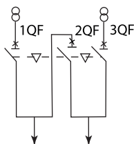
Рисунок 47. Блокировка трех автоматических выключателей
