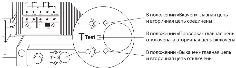
Рисунок 11. Индикатор положения выдвжной панели
