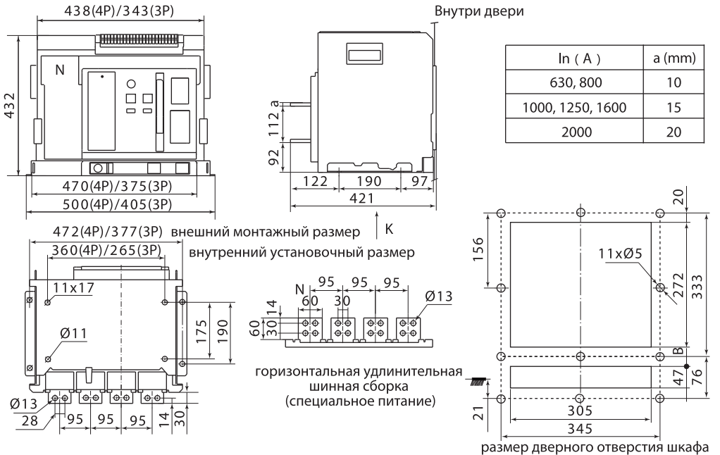
Рисунок 22. Габаритные и установочные размеры ВА90-2000 – выдвигное исполнение, мм
