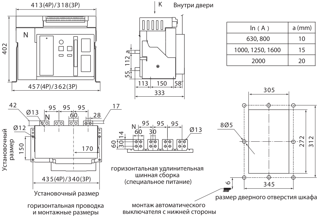
Рисунок 21. Габаритные и установочные размеры ВА90-2000 – стационарное исполнение, мм
