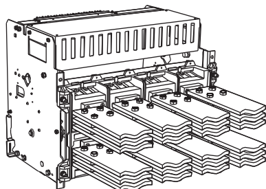
Горизонтальное подключение выше 1600 А с горизонтальной разводкой
