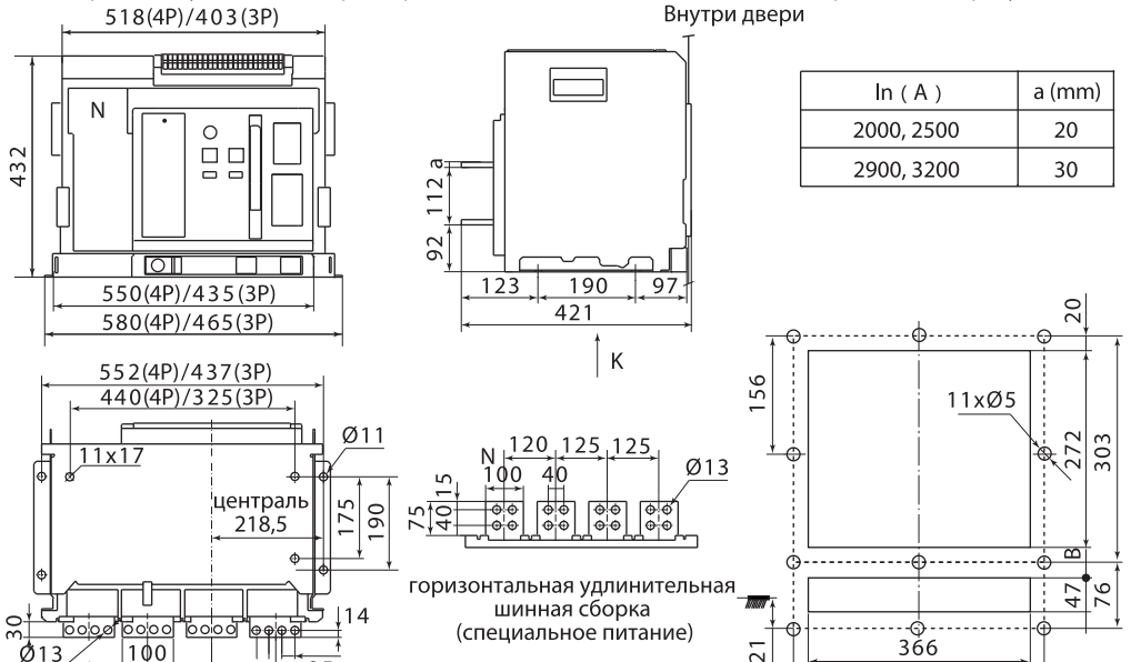
Рисунок 24. Габаритные и установочные размеры ВА90-3200 – выдвжное исполнение, мм
