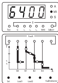
Рисунок 16. Настройка проверочного выключения
