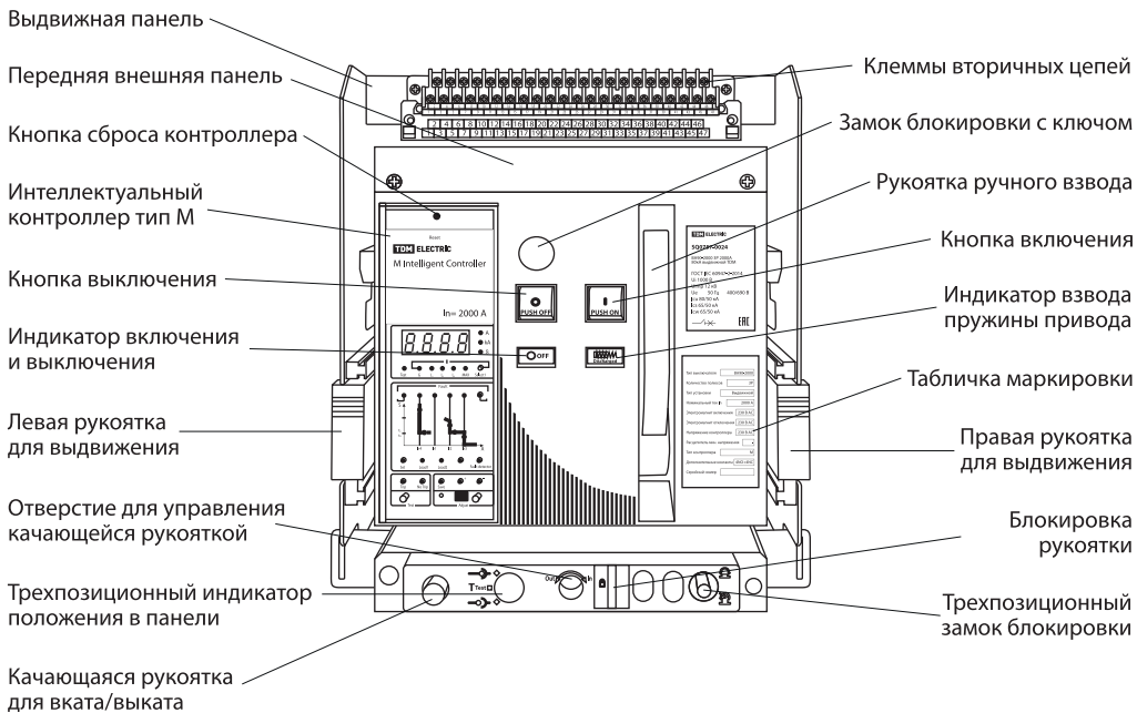
Рисунок 2. Автоматический выключатель выдвигного типа (пример, ВА90-2000)
