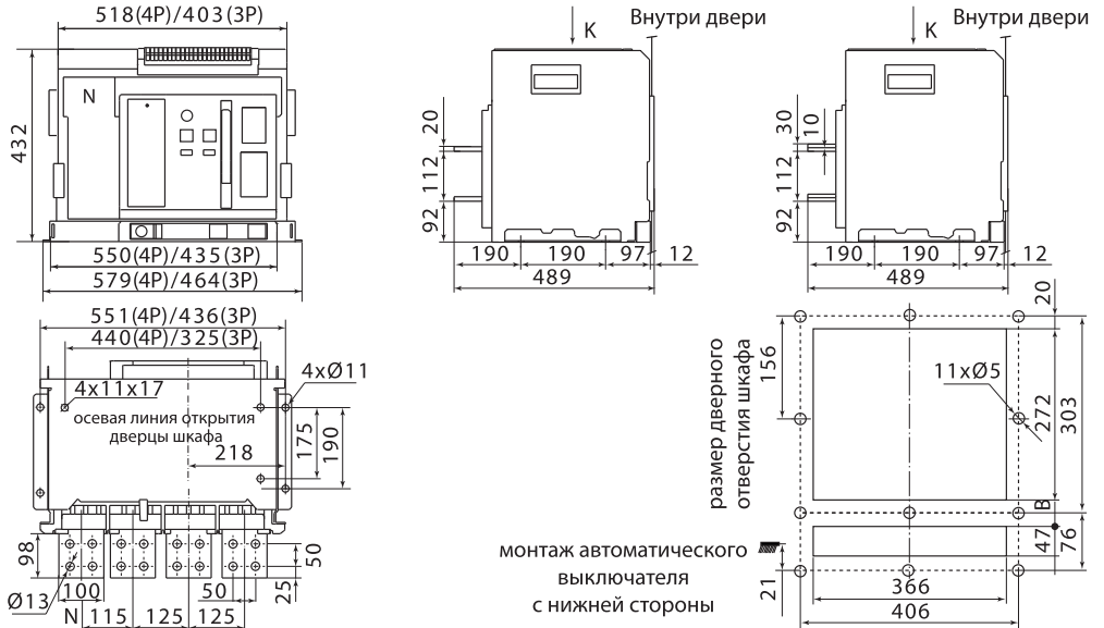
Рисунок 26. Габаритные и установочные размеры ВА90-4000 – выдвжное исполнение, мм
