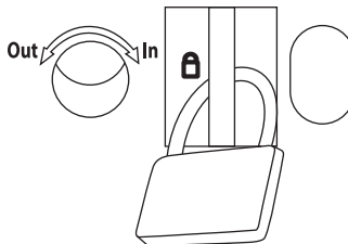
Рисунок 44. Запирание выдвижной панели на замок
