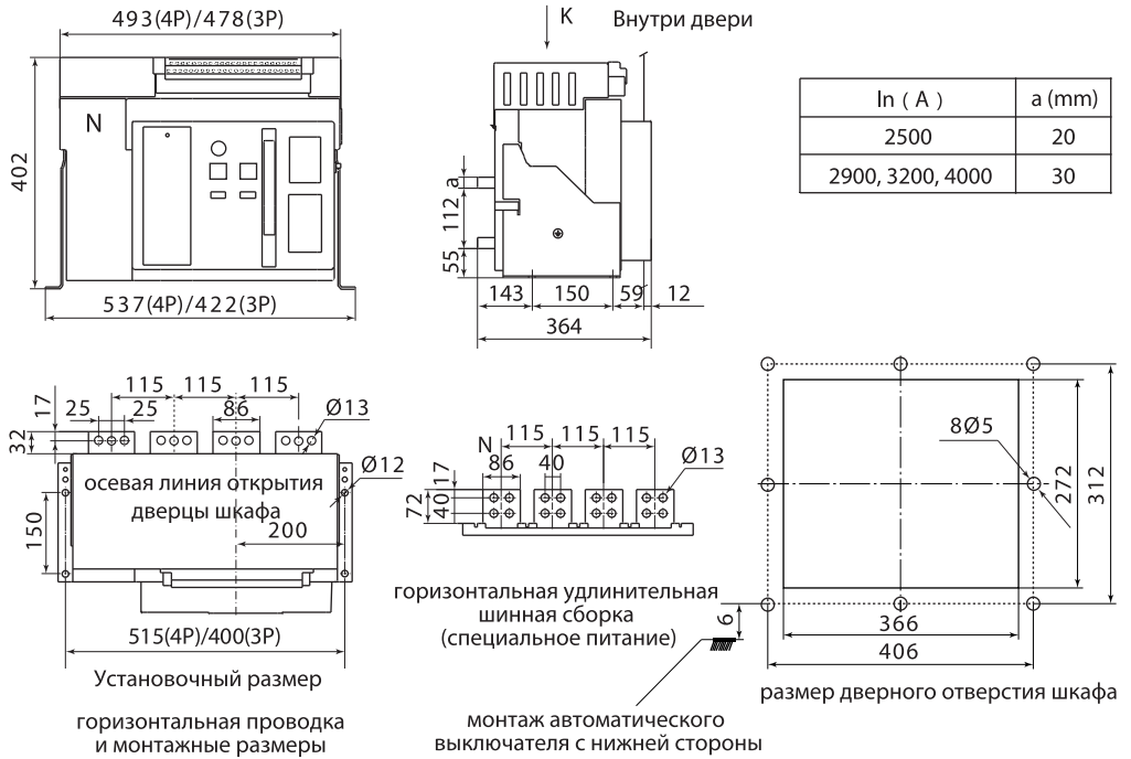
Рисунок 25. Габаритные и установочные размеры ВА90-4000 – стационарное исполнение, мм
