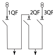
Рисунок 41. Метод 3: двухсторонняя блокировка питания двусторонней нагрузки
