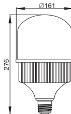
Рисунок 34 – Лампа LED-HP, 65 Вт, цоколь E40
