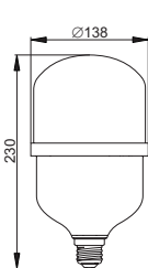
Рисунок 32 – Лампа LED-HP, 50 Вт, цоколь E27
