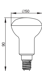
Рисунок 22 – Лампа LED–R50, 5 Вт цоколь E14
