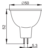
Рисунок 16 – Лампа LED–MR16, 3 Вт, 5 Вт цоколь GU5.3
