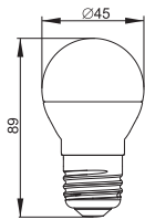
Рисунок 15 – Лампа LED–G45, 7 Вт, 9 Вт, цоколь E27
