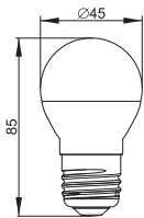
Рисунок 13 – Лампа LED–G45, 5 Вт цоколь E27
