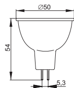
Рисунок 18 – Лампа LED–MR16, 9 Вт цоколь GU5.3
