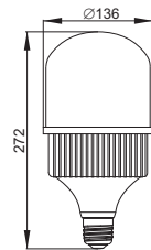
Рисунок 35 – Лампа LED-HP, 80 Вт, 100 Вт, цоколь E40
