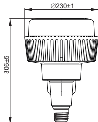
Рисунок 38 – Лампа LED- HP, 160 Вт, цоколь E40
