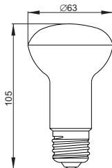
Рисунок 23 – Лампа LED–R63, 5 Вт, 8 Вт цоколь E27
