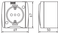
Рис. 1 - Габаритные размеры 1-местной розетки
