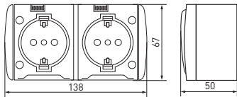
Рис. 2 - Габаритные размеры 1-местной розетки
