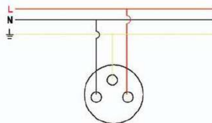
Схема цепи / Wiring Diagram
