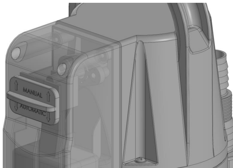
Рисунок 5 – Переключатель режима работы насоса
