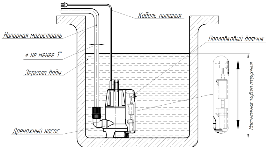
Рисунок 6 – Пример размещения насоса в скважине
