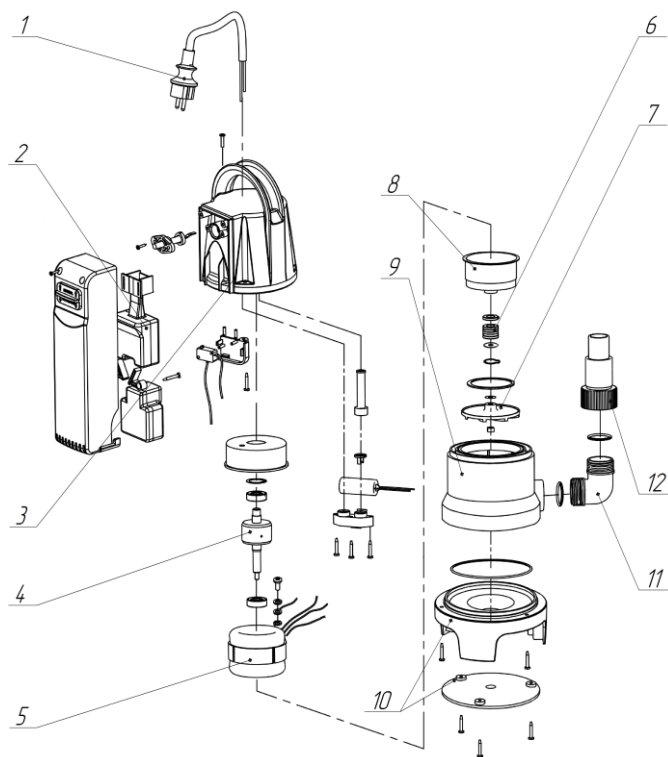
Рисунок 3 – Общий вид и конструкция насоса для грязной воды
