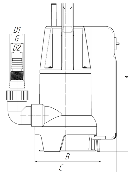
Рисунок 4 – Габаритные и присоединительные размеры изделия
