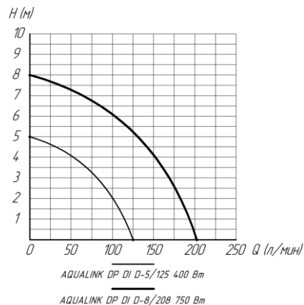
Рисунок 2 – График зависимости показателей напорно-расходных характеристик насосов для грязной воды, H – напор; Q – расход.
