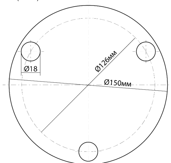
Рис. 1 Основание светильника
