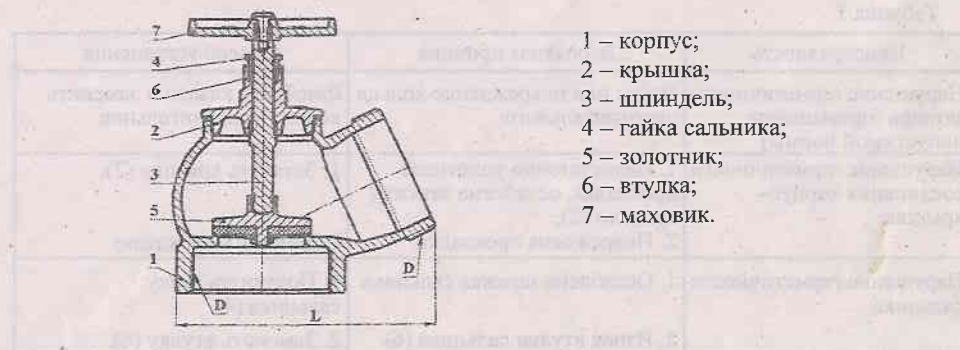
Рисунок 1. Клапан ПК ч, м-ц
