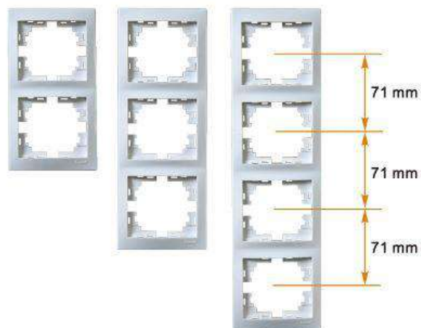
Рамка вертикальная / Vertical Frames
