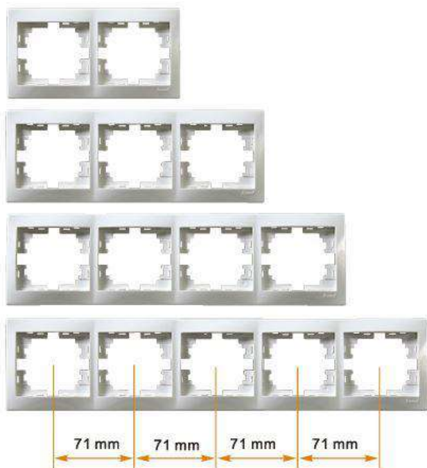
Рамка горизонтальная / Horizontal Frames
