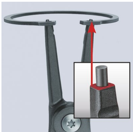
Щипцы KNIPEX прецизионные для стопорных колец: не деформируют кольца, легкий и быстрый монтаж
