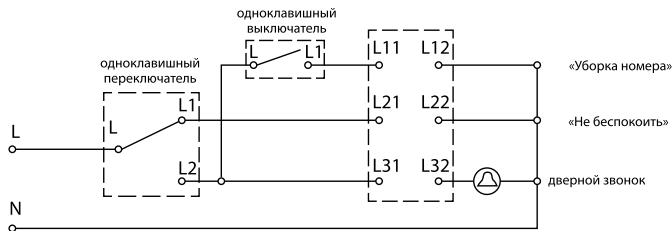
Рисунок 1. Схема подключения
