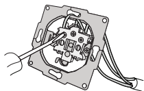
3.3. Присоединить провода, вставив зачищенные концы в пазы контактных зажимов, затянув винты.
