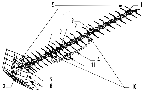
Рис.1 Общий вид антенны
