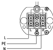
Единичное подключение
