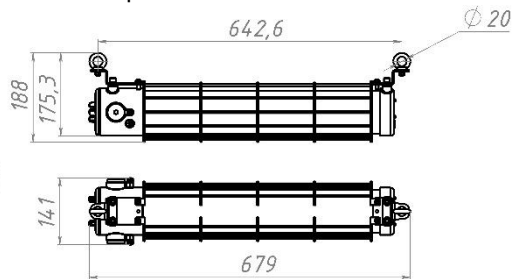
На рым-болтах
