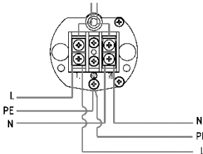
Транзитное подключение
