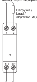
Рисунок 4 – Схема подключения реле с типом выходного напряжения А и наличием встроенного радиатора / Figure 4 – Wiring diagram of relay with output voltage type A and built-in radiator / 4 сурет – А шығыс кернеуі типімен және ендірмелі радиатормен бірге SSR1 релені жалғау схемасы
