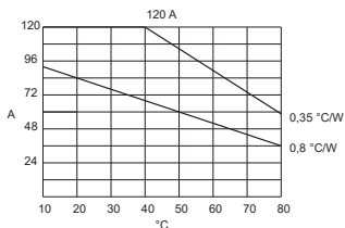
Рисунок 6 – Графики зависимости номинального тока реле от температуры окружающей среды с типом цепи управления А и D / Figure 6 – Graphs of relay rated current dependence on ambient temperature with control circuit type A and D / 6 сурет – Басқару тізбегінің типі А және D реленің номиналды тогының қоршаған ортаға тәуелділік графикатері
