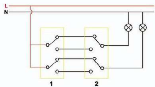
Схема цепи / Wiring Diagram
