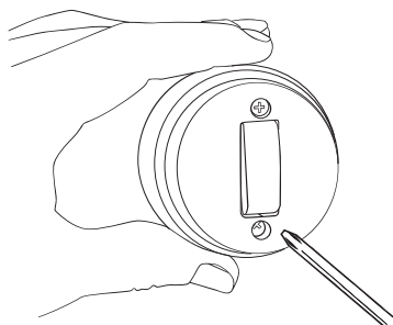
Рисунок 1. Вывернуть два самореза и снять корпус изделия.
