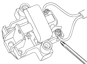
Рисунок 2. Прикрепить корпус изделия к стене двумя шурупами (в комплект не входят). Зачищенные провода вставить в контакты. Затянуть винты клемм.
