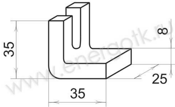
Контакты к контакторам (подвижные) КТ6033
