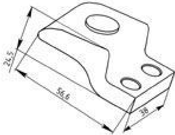
Контакты к контакторам (подвижные) КТ6053
