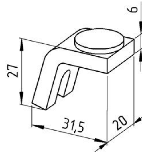
Контакты к контакторам (неподвижные) КТ6633
