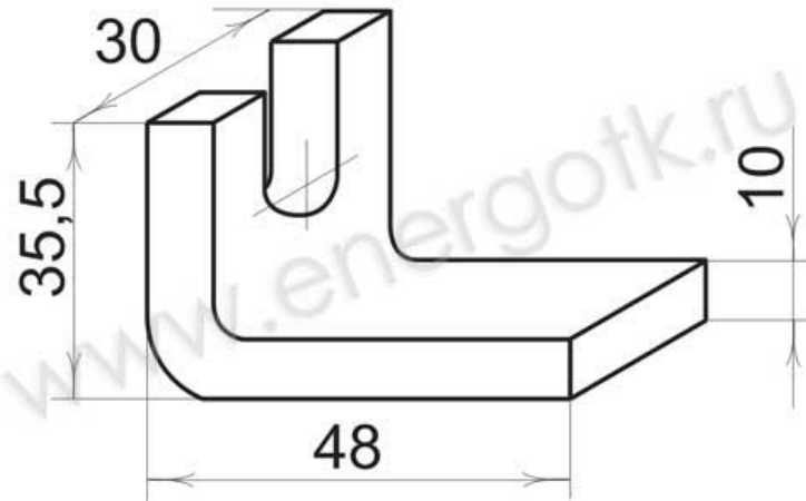
Контакты к контакторам (неподвижные) КТ6043
