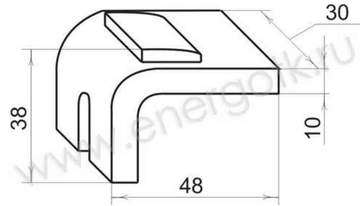
Контакты к контакторам (неподвижные) КТ6033С
