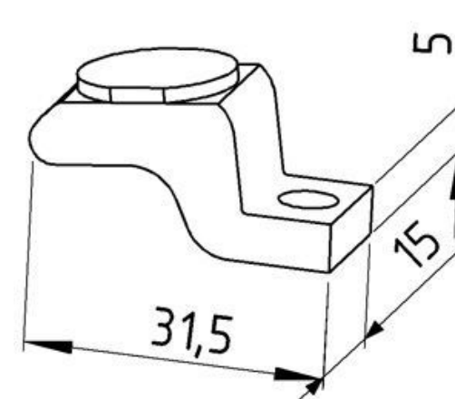
Контакты к контакторам (подвижные) КТ6633
