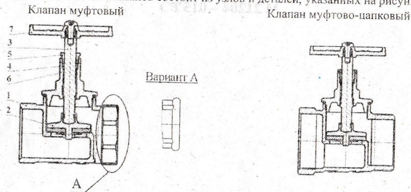
Рисунок 1 – Клапан запорный
