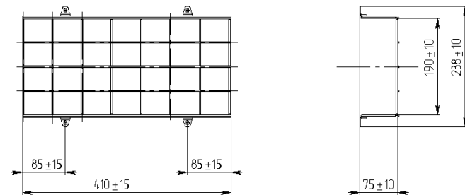
Сурет 1. Қорғаныс торын орнату схемасы
