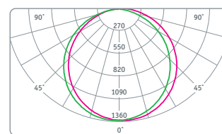
DPO-02-36-4K-IP20-LED CRI90
