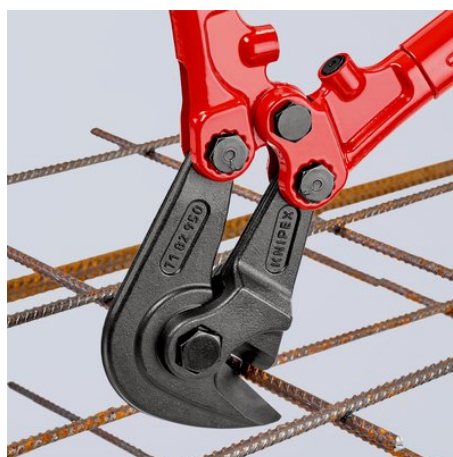
Особая форма головки ножниц для резки арматурной сетки 71 82 950 позволяет резать плотно прилегающую арматуру
