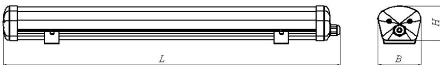
Рис. 1. Общий вид светильников серии Luxe
