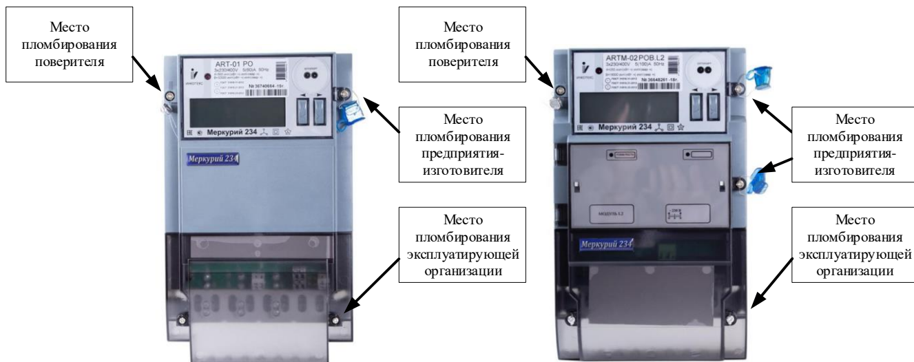
Рисунок 3.5 – Общий вид счетчиков «Меркурий 234» с указанием мест пломбирования и нанесения знака поверки
