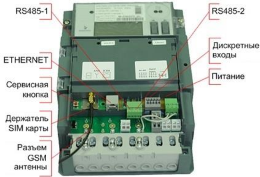
Рисунок 5.6 Элементы подключения модуля телемеханики
