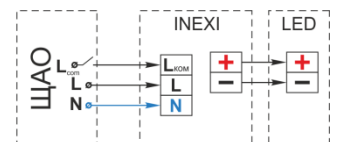
группы LCGt
