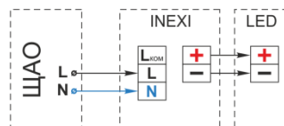
группы Bt
