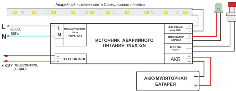
Рис. 2 Схема подключения BS-INEXI2-81-B2-LED и BS-INEXI2-83-B2-LED для аварийного светового прибора в непостоянном режиме:
