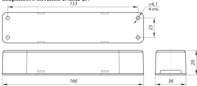
Рис.7 Габаритные и присоединительные размеры источника аварийного питания INEXI-2N
