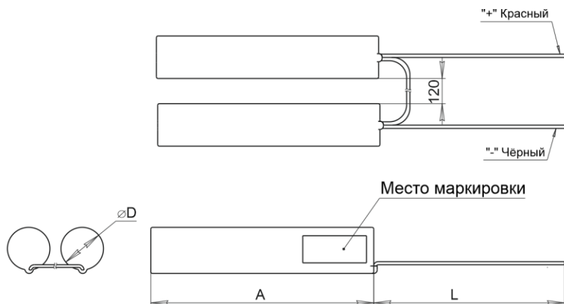
Рис.10 Габаритные размеры АКБ BS-2+2KRHT23/43-1.5/L-HB500-0-1 а18266
