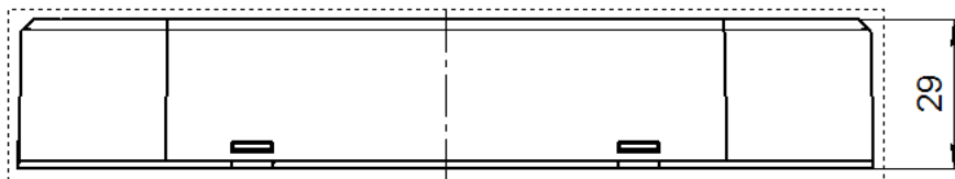
Рис.7 Габаритные и присоединительные размеры источника аварийного питания INEXI N
