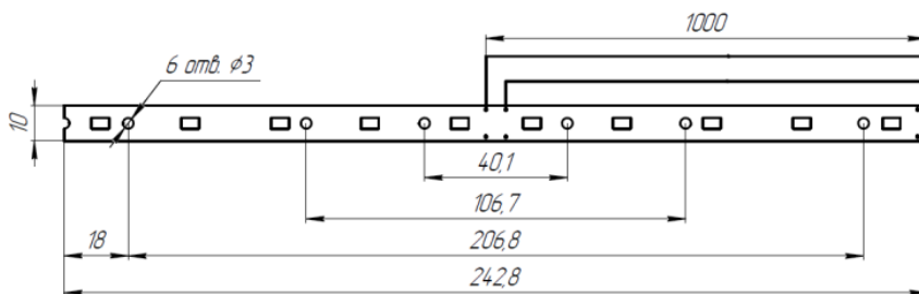
Рис.8 Габаритные и присоединительные размеры светодиодной линейки BS-LED-C01-100-5000 а29543
