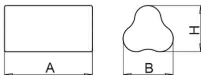
Рис.10 Габаритные размеры АКБ BS-2+2KRHT23/43-1.5/L-HB500-0-1 а18266
