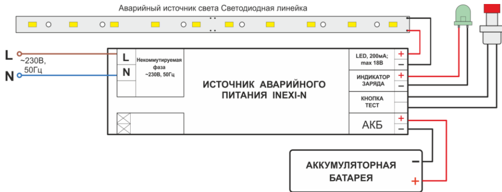
Рис. 2 Схема подключения BS-81-B1-LED и BS-83-B1-LED для аварийного светового прибора в непостоянном режиме:
