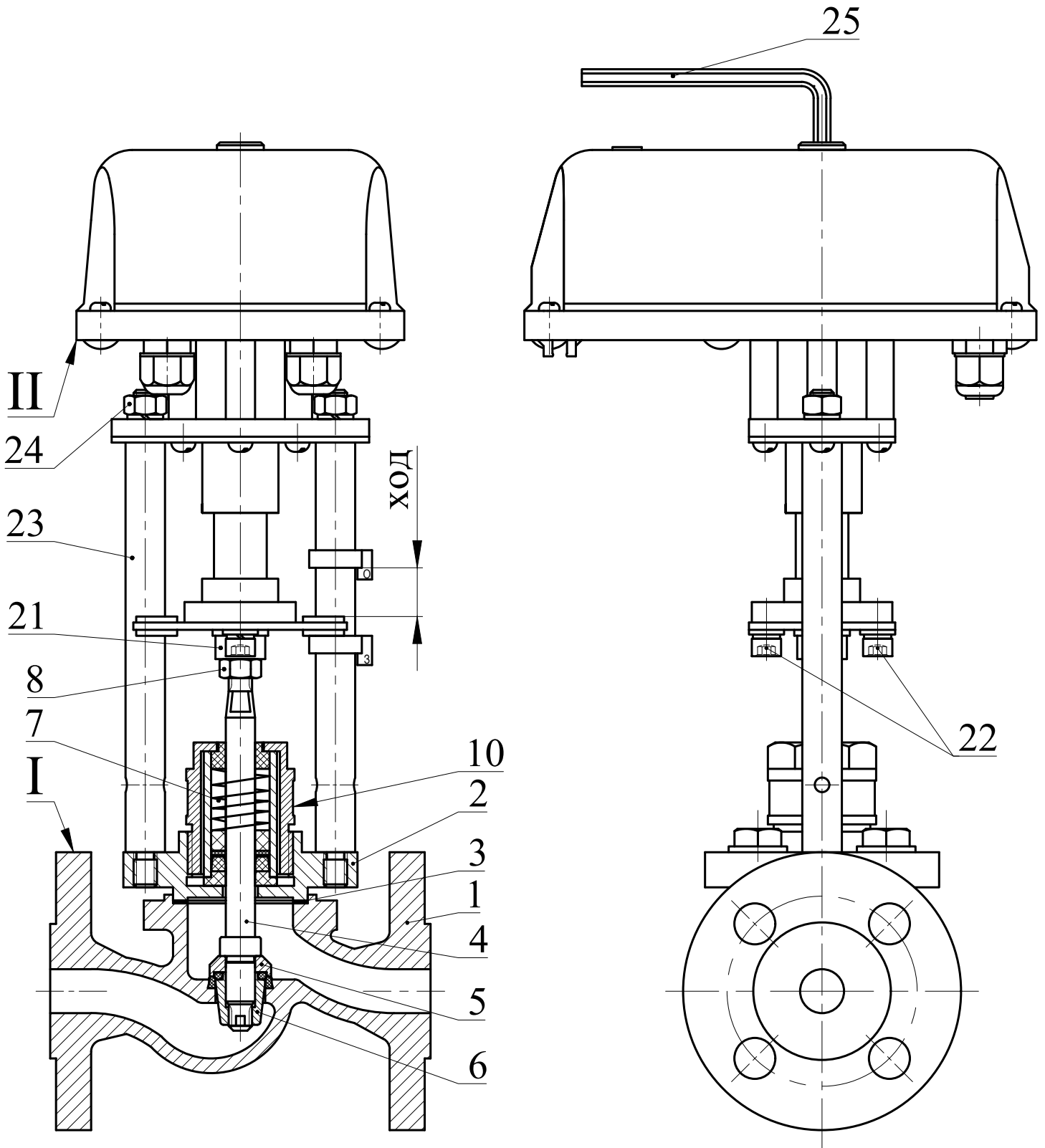
Рисунок 2 - DN15, Kvу 0,63 - 4,0 DN20 - DN50
