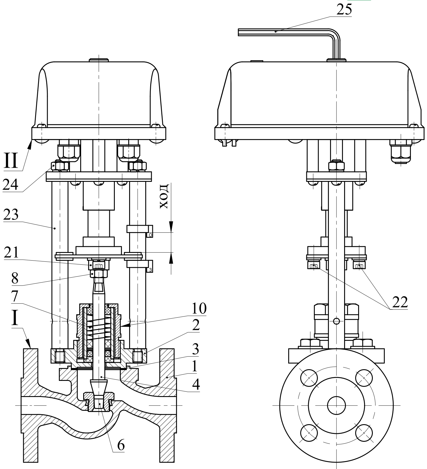
Рисунок 1 - DN15, Kvу 0,25; 0,4
