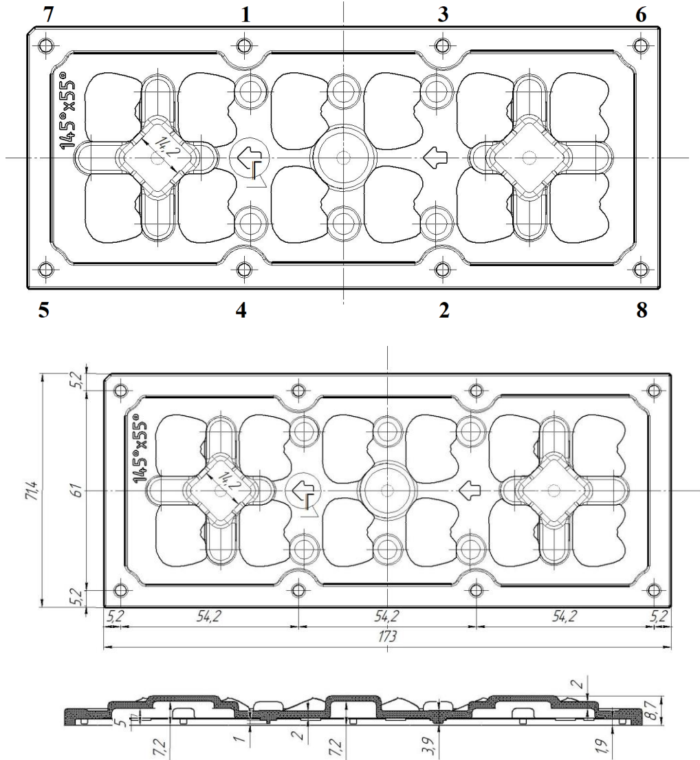
Чертёж линзы
