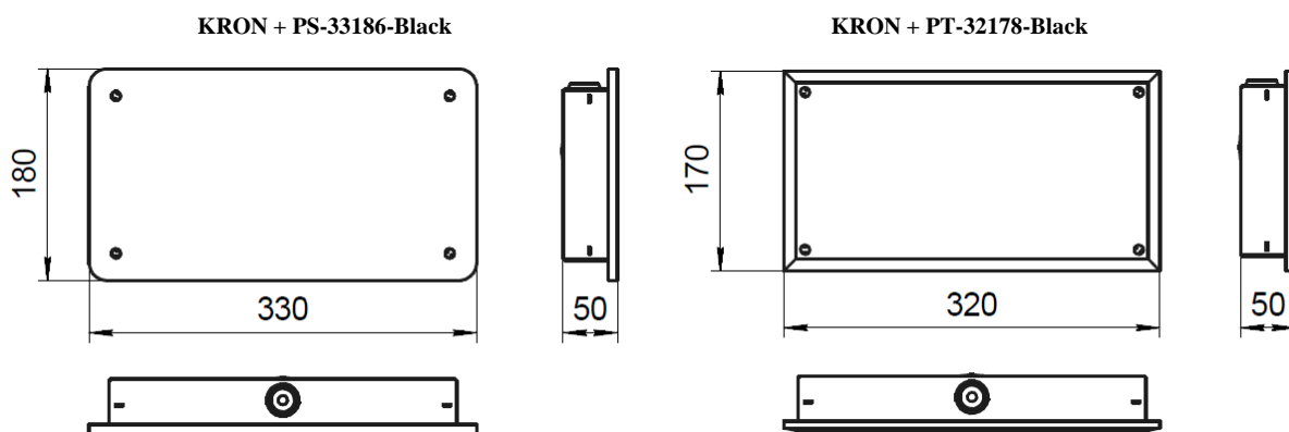
Рис. №2 Габаритный чертёж.
