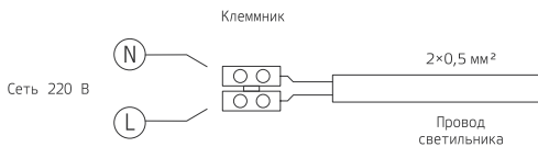
Рис. 1. Схема подключения светодиодного светильника INDUSTRY к сети 220 В
