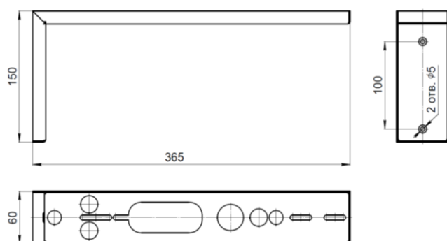
Рис. №7 Аксессуары. Кронштейн BS-K-3
