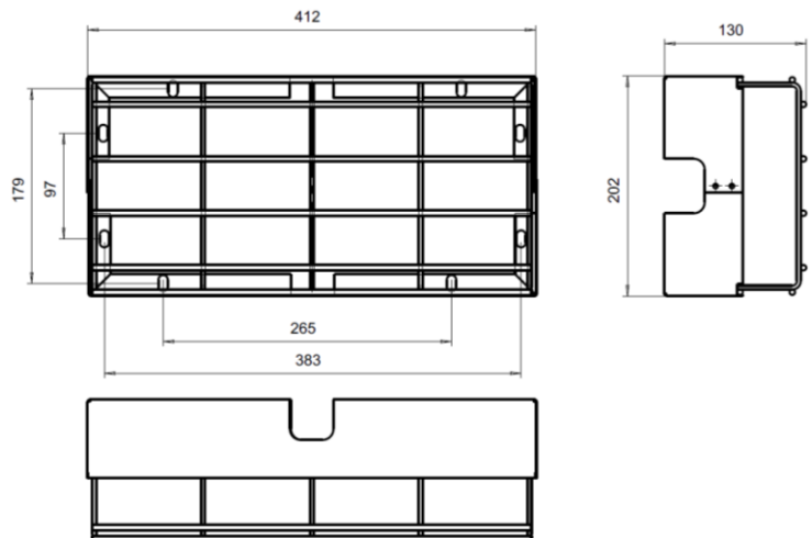
Рис. №6 Аксессуары. Решётка защитная BS-R-1 (a2333)
