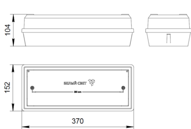
Рис. №5 Габаритный чертёж.
