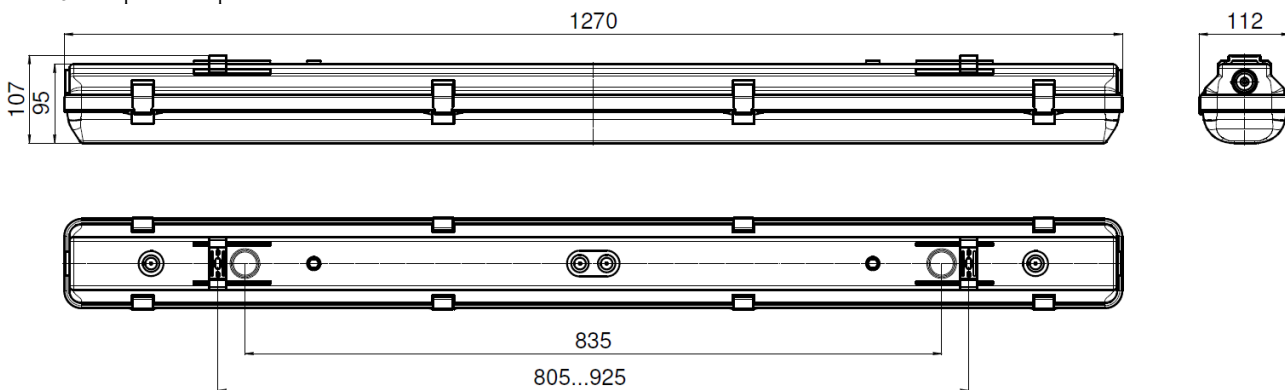
Рис. №5 Габаритный чертёж
