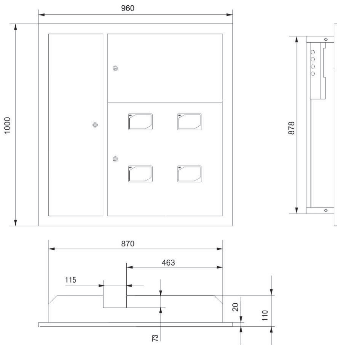
Рисунок 1 – Корпус на 2–6 квартир
