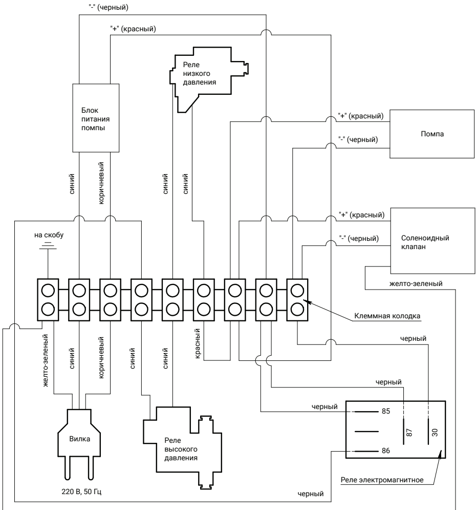
Рис. 14 Электрическая схема.
