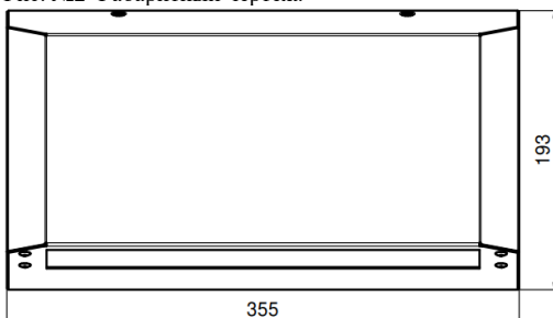
Рис. №2 Габаритный чертёж.
